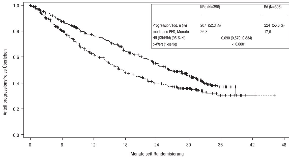
Abbildung 1: Kaplan-Meier-Kurve des progressionsfreien Überlebens bei rezidiviertem multiplen Myelom a
