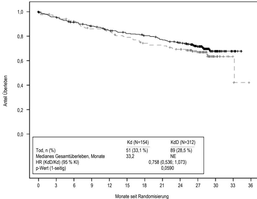
Abbildung 6: Kaplan-Meier-Kurve des Gesamtüberlebens in Studie 20160275
